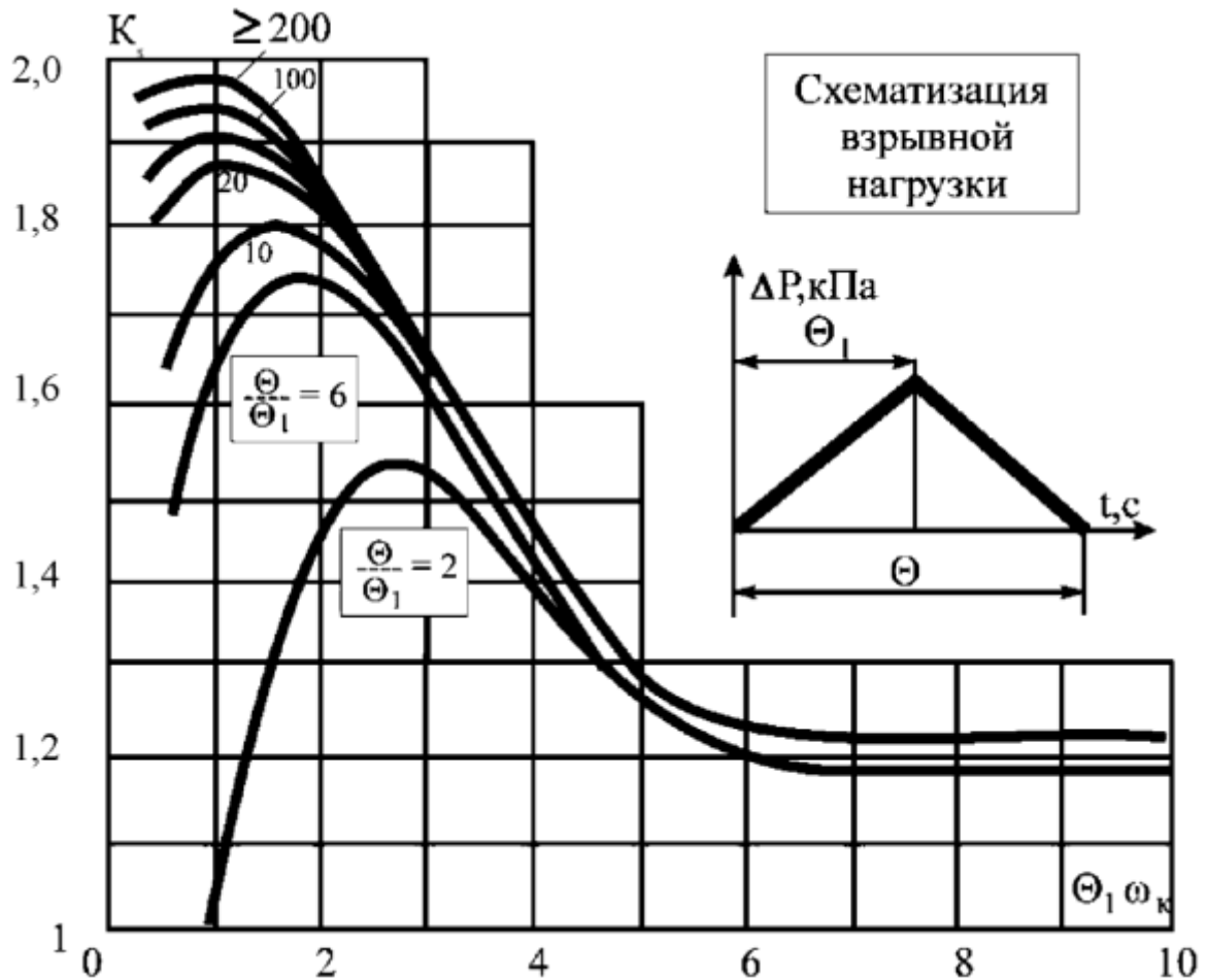
Рисунок 7.1 - График для определения коэффициента динамичности K_d
