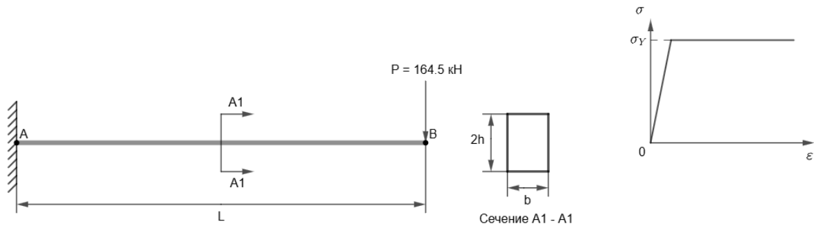
Рисунок 1 – Расчетная схема
