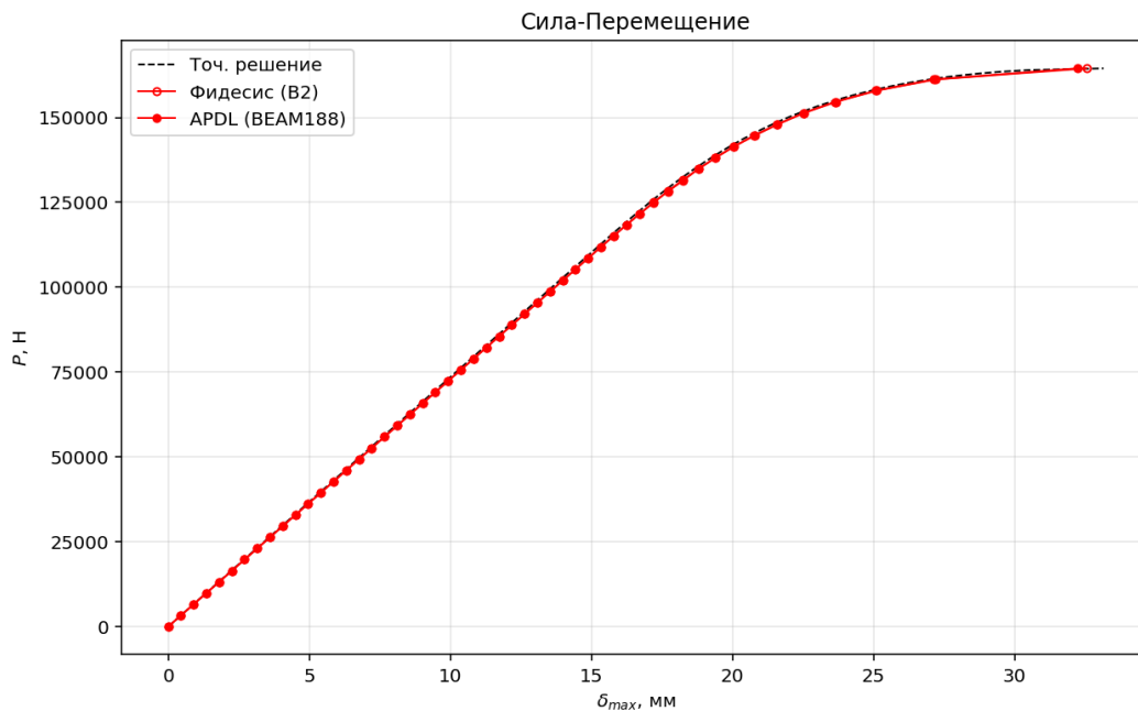
Рисунок 3 – Кривые Сила-Перемещение
